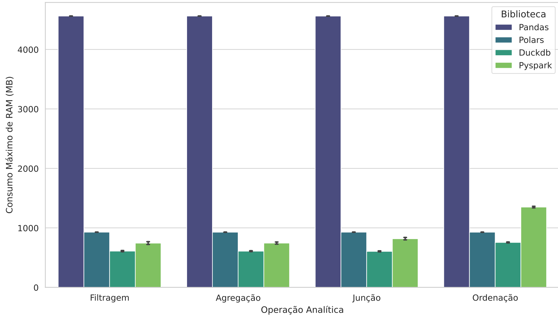
Consumo de RAM Pico (MB) por Operação - Dataset 512MB
