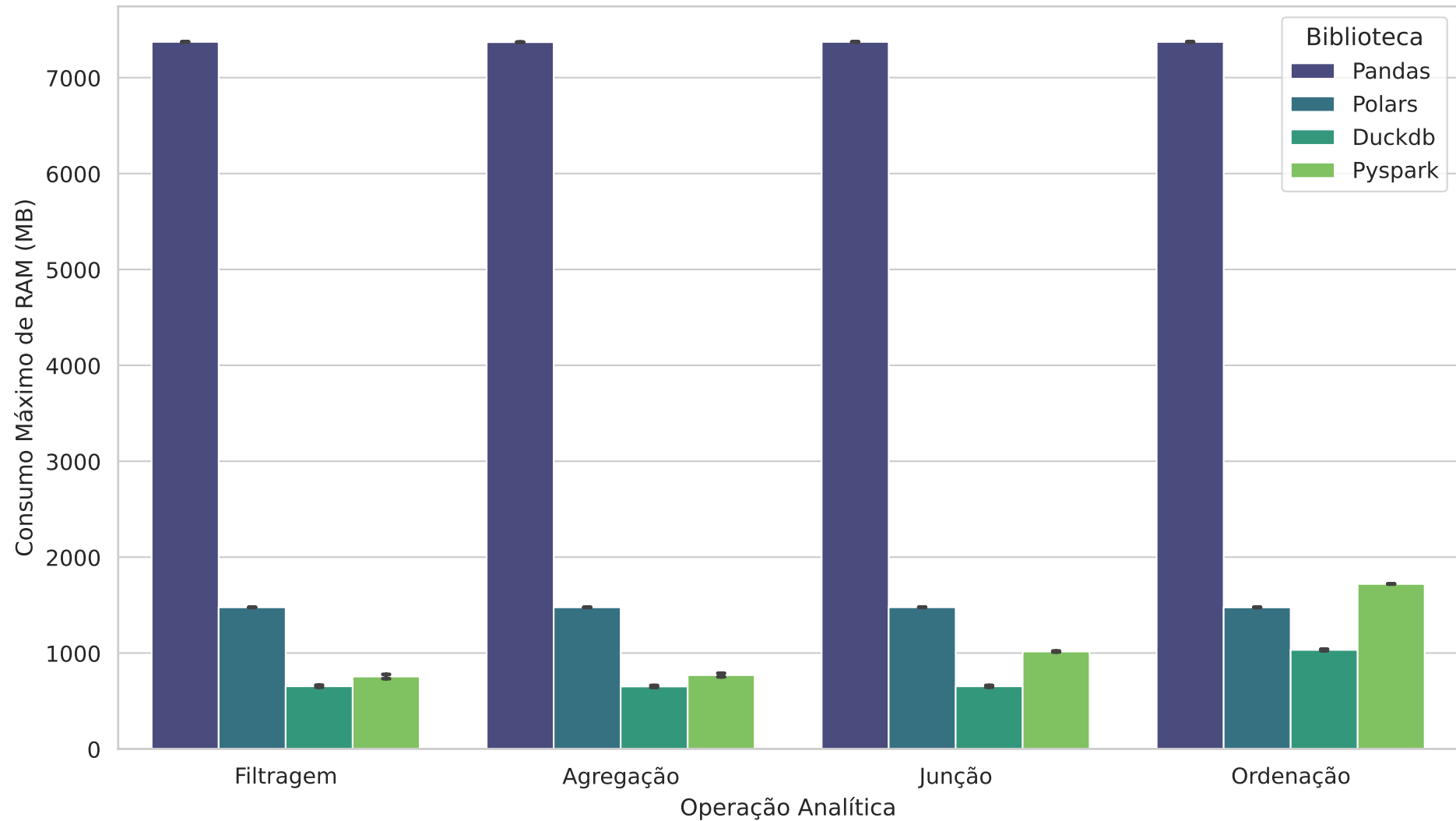
Consumo de RAM Pico (MB) por Operação - Dataset 1024MB
