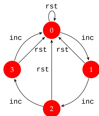
Slika 1: Dijagram prelaza dvobitnog brojača. Brojač podržava spoljne komande „inkrementiraj se” (inc) i „resetuj se” (rst).
