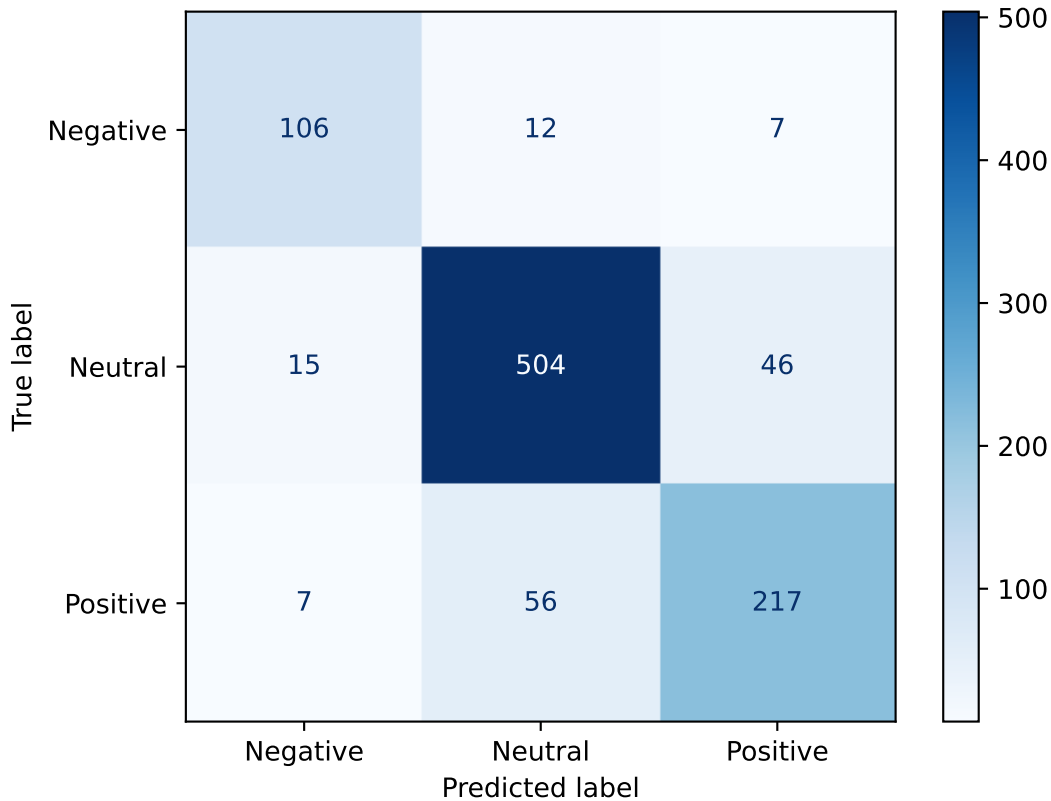
Confusion Matrix — Financial Sentiment (BERT)
