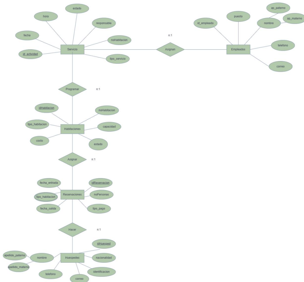
Imagen 2. Diagrama de Entidad-Relación (DER)
