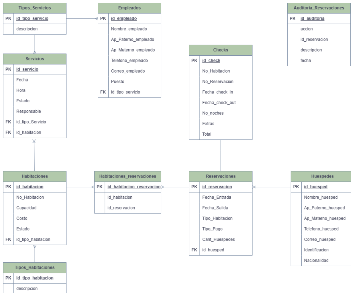
Imagen 3. Diagrama relacional normalizado
