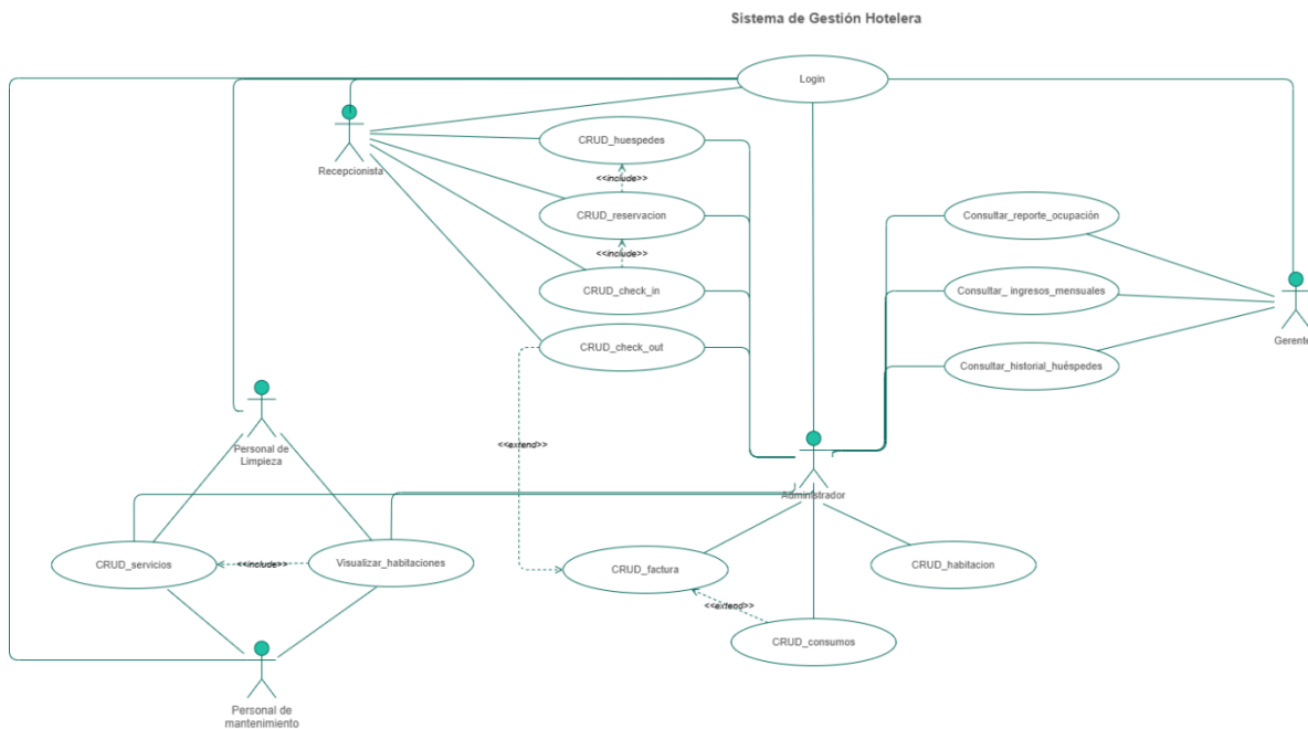
Imagen 1. Diagrama de casos de uso y roles del sistema (Administrador, Recepcionista, Limpieza y Gerente).
