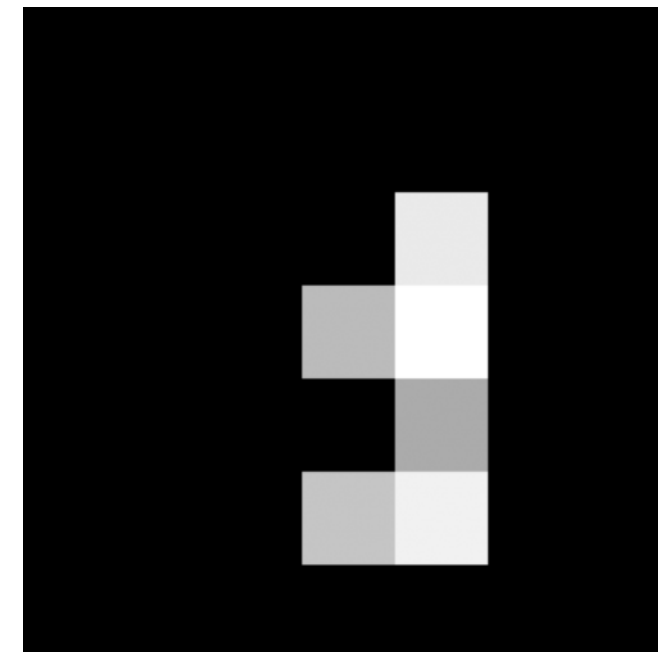
Grad-CAM mask)
