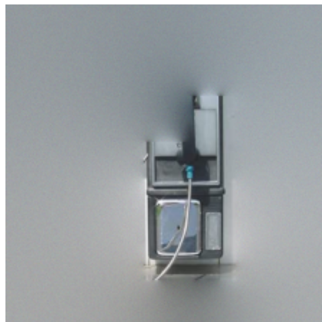
LeRF (Linear)
