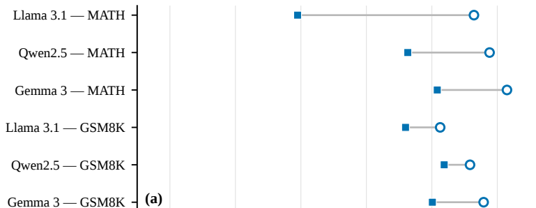
Raw MLP
