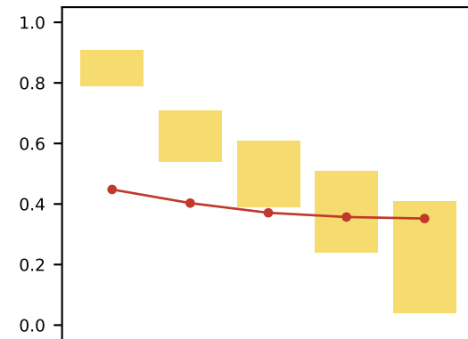
S2, beta 1
