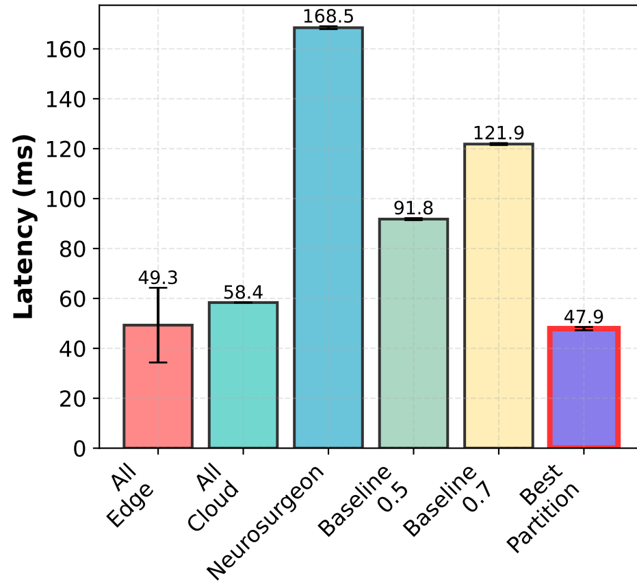
(b) VGG-11
