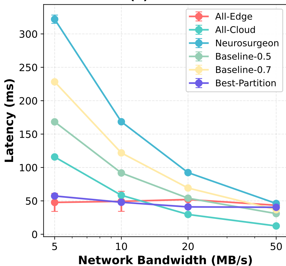
(b) VGG-11
