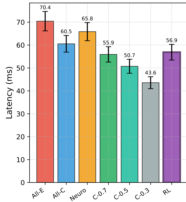
VGG-16
