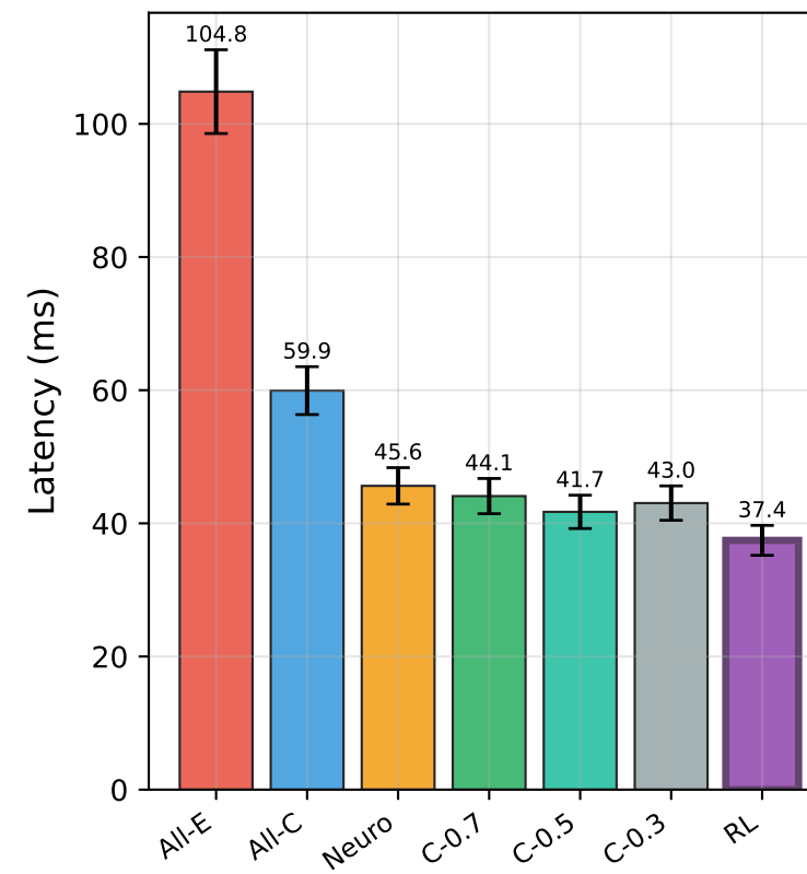
MobileNet-V2
