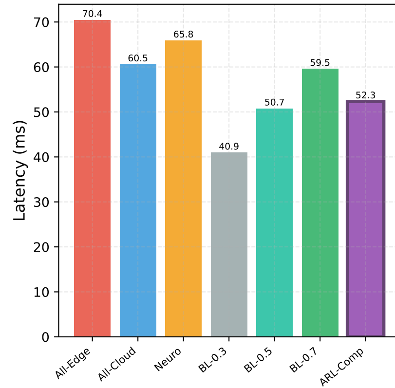
VGG-16
