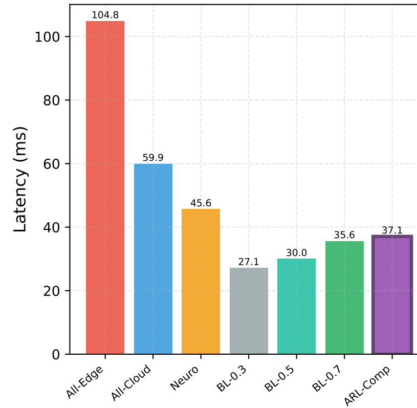
MobileNet-V2
