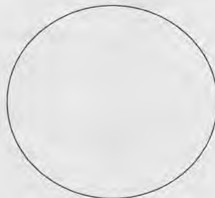
Пустое множество
