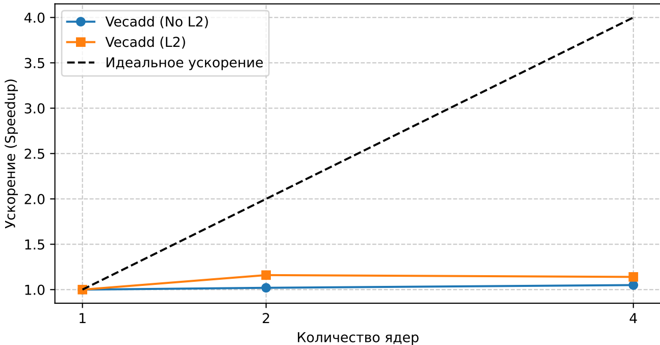
Strong Scaling: Ускорение vs Ядра (Vecadd - Memory-Bound)
