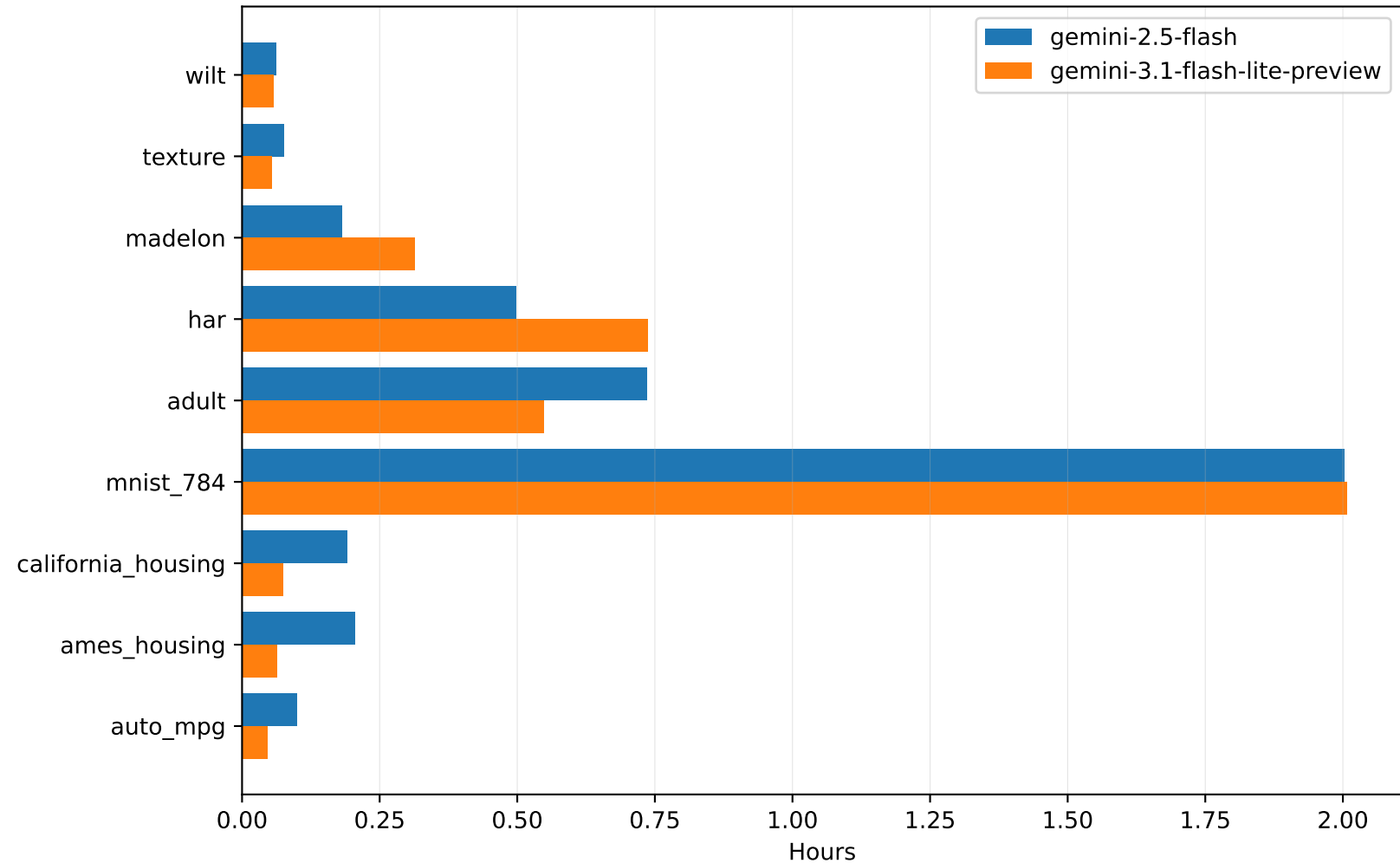
Actual wall-clock time by dataset
