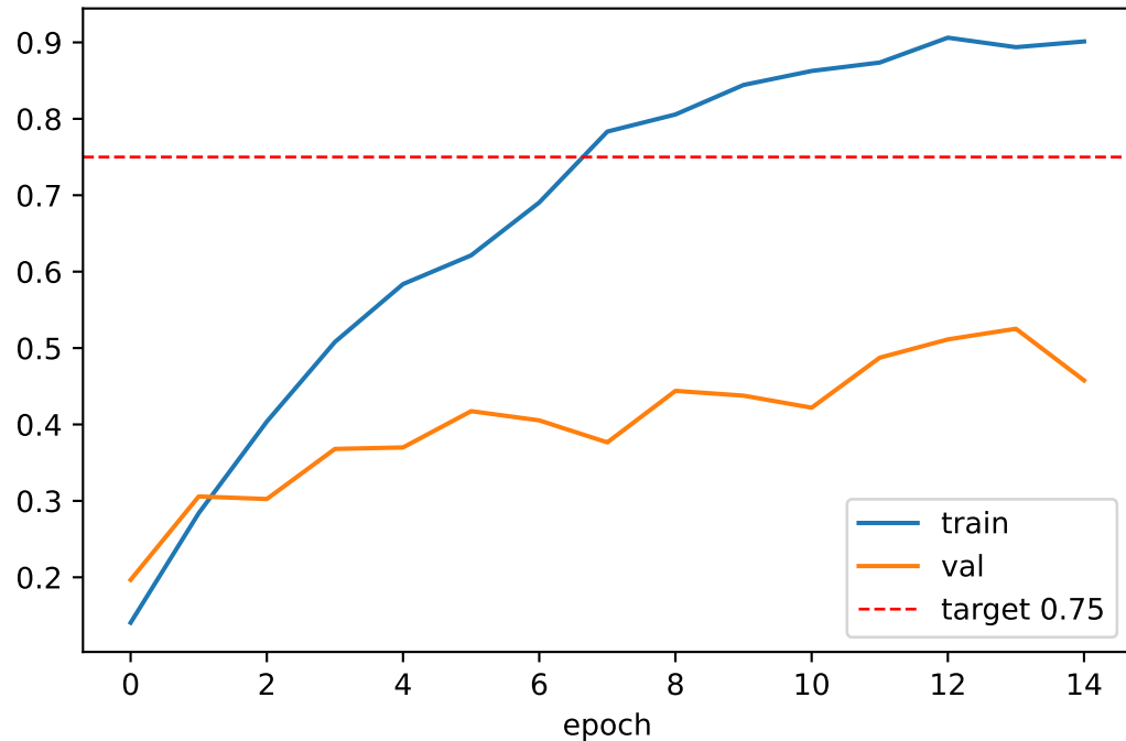
BiRNN - Macro F1
