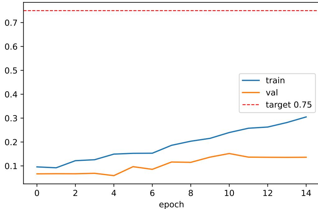
Vanilla_RNN - Macro F1
