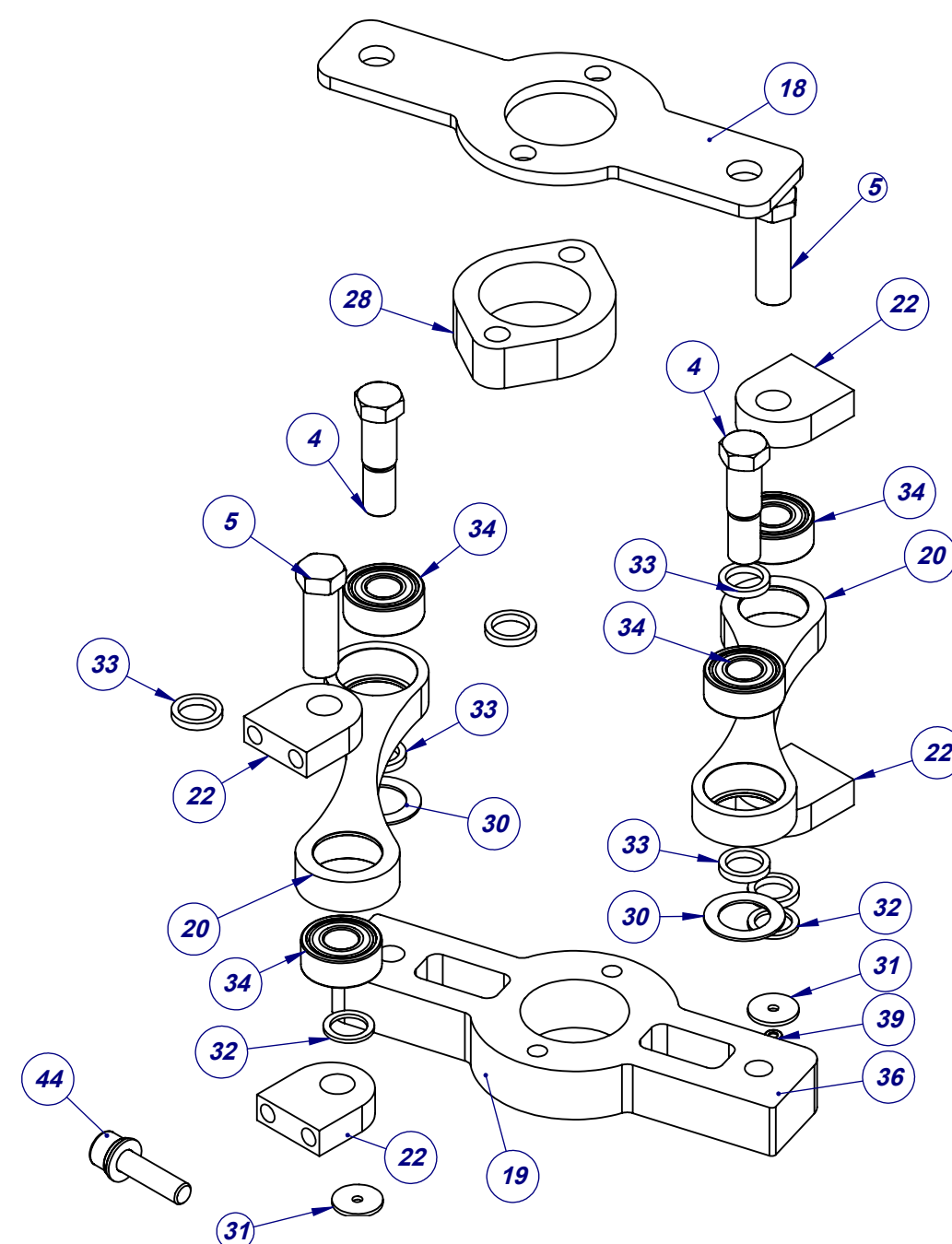
Cotas críticas de inspeção ( ) Cotas apenas para referência Rugosidade: _____ Cliente: _____ Nº Des.: _____ Denominação: CJ QUADRO ABRE FECHA SERVO AB VPL - RED.SEW 1/29 Insumo: 250011 Revisão: 01 Revestimento: - Folha: 2 / 3 Escala: 1:8 Peso (kg): 95.08 Unidades: mm Formato: A2 RAUMAK PACKAGING Proj.: Lucas B. Novack Des.: Lucas B. Novack Aprov.: Ademar Rutke Data: 23/04/2024 Este documento é de propriedade da Raumak Máquinas, sendo proibida sua reprodução total ou parcial, bem como sua divulgação sem autorização prévia. Obs.: Caso o campo "N" des. "estiver em branco, considerar o código do campo "Insumo".
