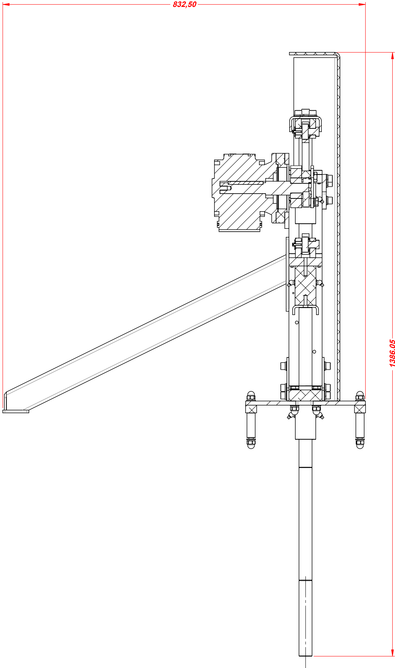
SEÇÃO A-A
