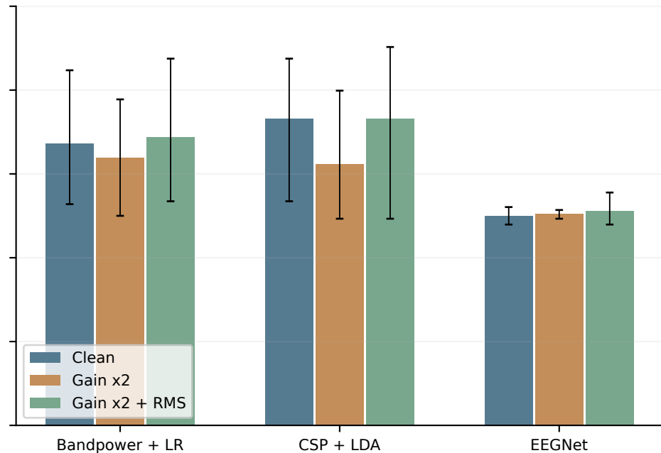
BNCI2014 001
