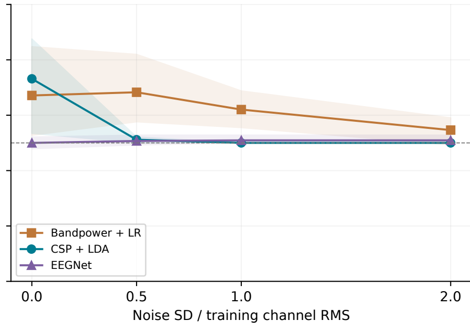
BNCI2014 001
