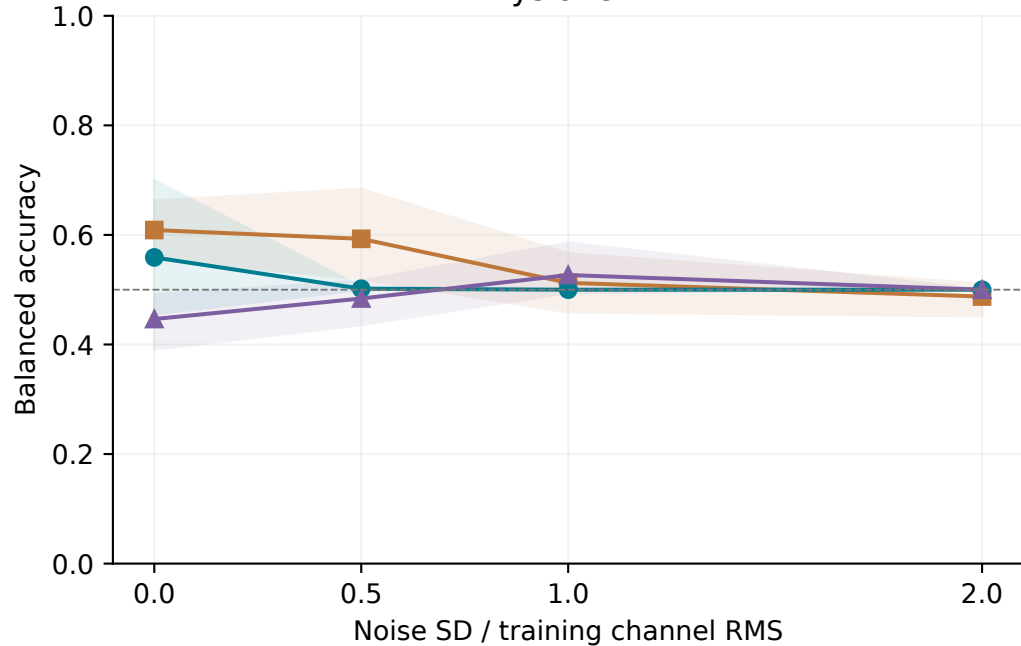
PhysionetMI
