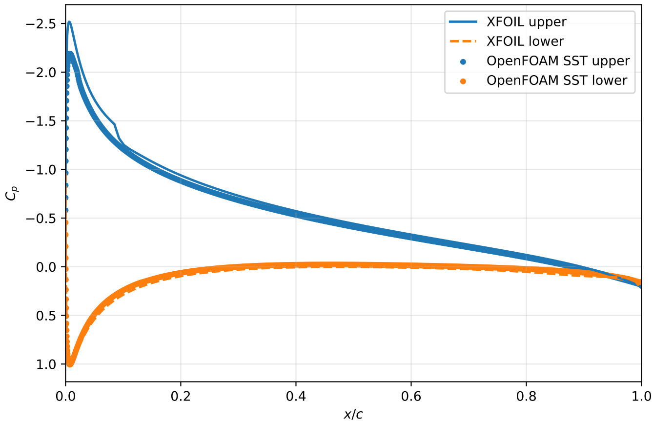
NACA0012, Re = 10^6 , AoA = 6^\circ
