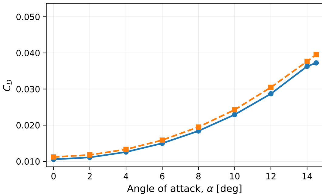
(a) NACA 0012
