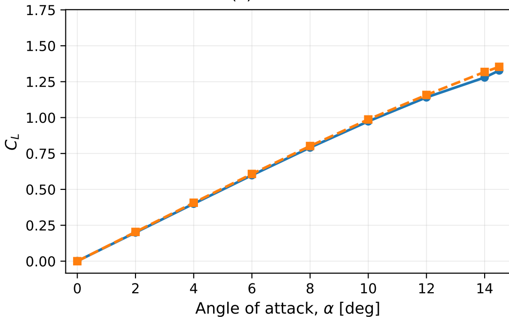
(a) NACA 0012
