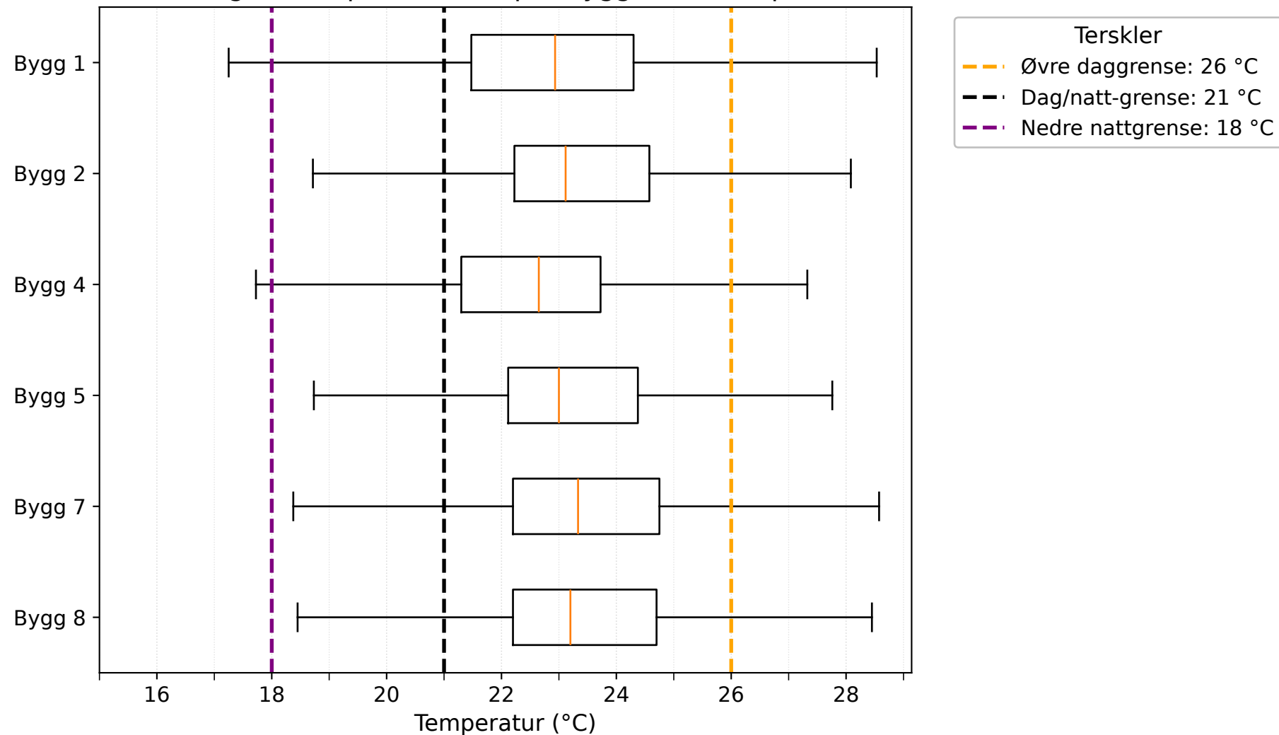
Fordeling av Temperatur (°C) per bygg hele måleperioden
