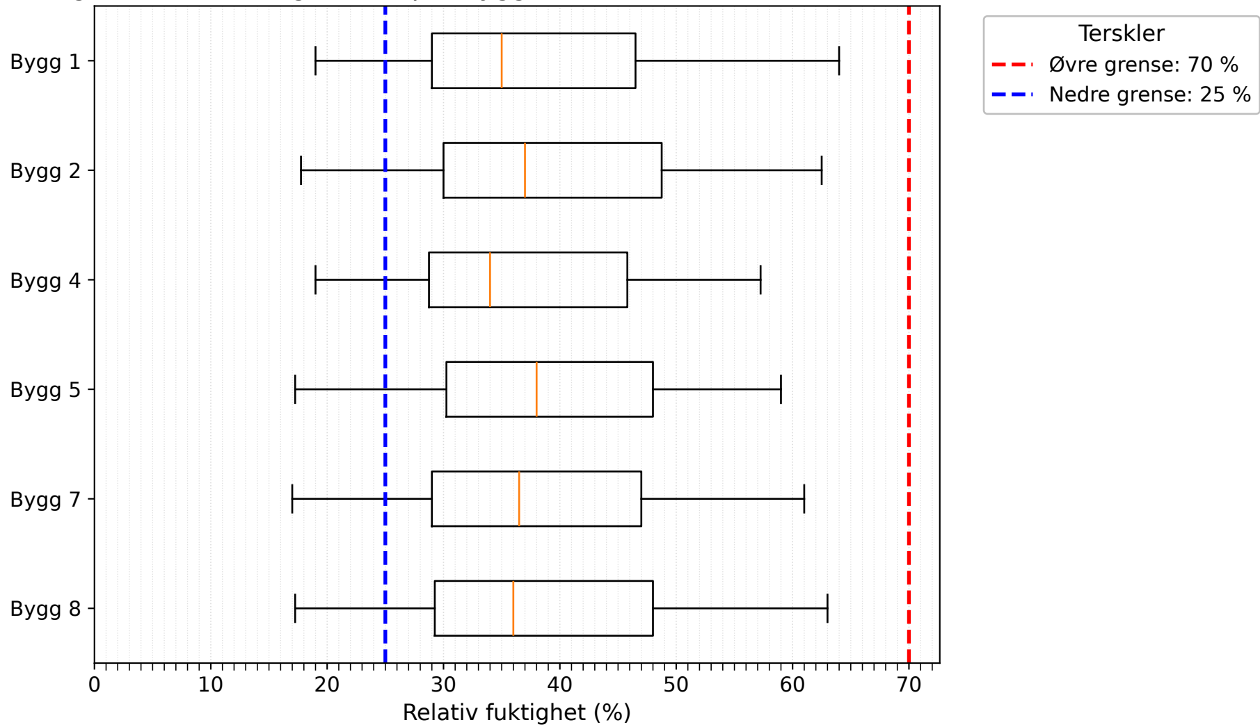
Fordeling av Relativ fuktighet (%) per bygg høsten 2023 (10.08.2023 til 10.12.2023)
