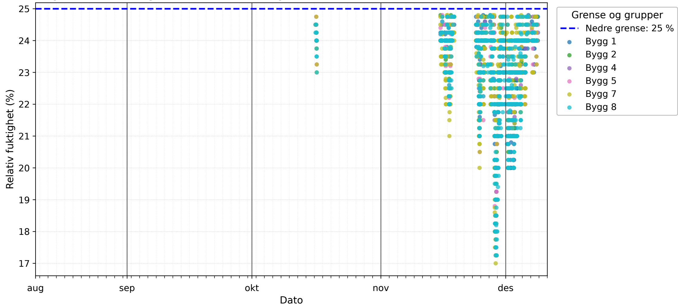
Målinger under nedre grense for Relativ fuktighet (%) høsten 2023 (10.08.2023 til 10.12.2023)
