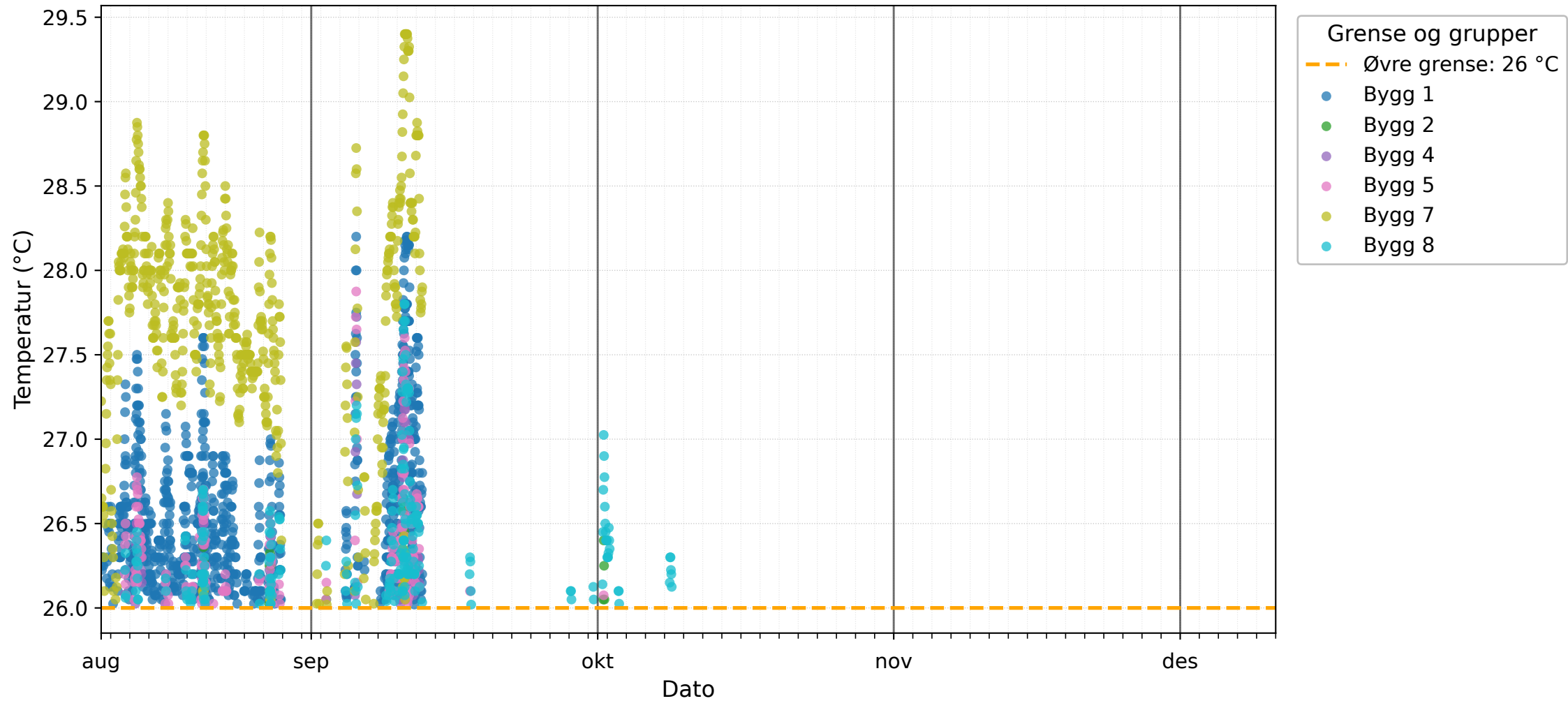
Målinger over øvre grense for Temperatur (°C) høsten 2023 (10.08.2023 til 10.12.2023)
