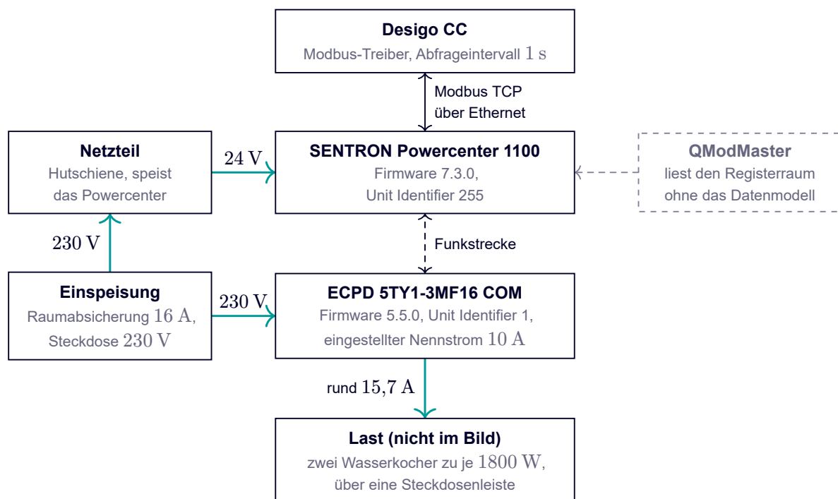
Abbildung 6: Verschaltung des Testaufbaus mit Einspeisung und Laststrom, der Funkstrecke zwischen ECPD und Powercenter, der Modbus-Anbindung an Designo CC über Ethernet sowie dem unabhängigen Modbus-Werkzeug zur Gegenprobe
