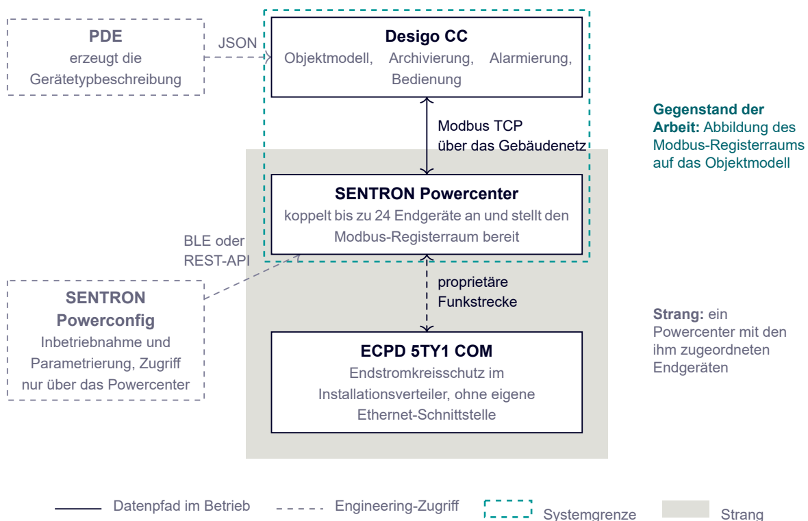
Abbildung 3: Datenpfad vom ECPD über die Funkstrecke zum Powercenter, von dort über Modbus TCP im Gebäudenetz zu Designo CC, seitlich angetragen die Werkzeuge SENTRON Powerconfig und PDE mit ihren jeweiligen Zugriffspunkten
