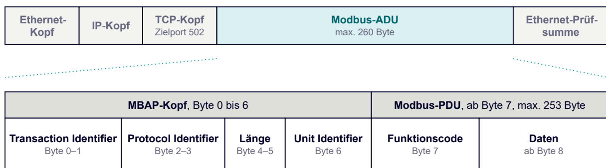
Abbildung 1: Aufbau eines Modbus-TCP-Telegramms, oben die Kapselung im Ethernet-Rahmen, unten die Felder der Anwendungsdateneinheit aus MBAP-Kopf und Protokolldateneinheit mit ihren Bytepositionen, die Feldbreiten sind nicht maßstäblich [13], [20]
