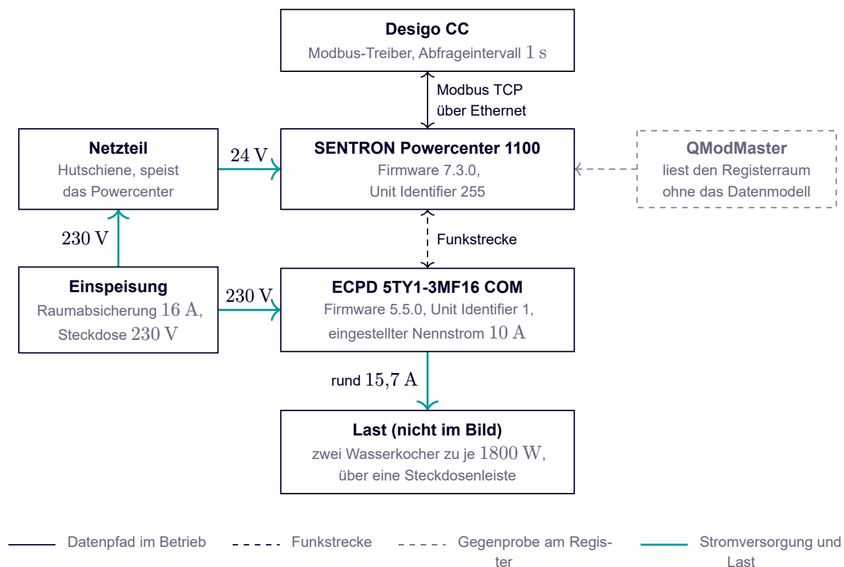
Abbildung 6: Verschaltung des Testaufbaus mit Einspeisung und Laststrom, der Funkstrecke zwischen ECPD und Powercenter, der Modbus-Anbindung an Desigo CC über Ethernet sowie dem unabhängigen Modbus-Werkzeug zur Gegenprobe
