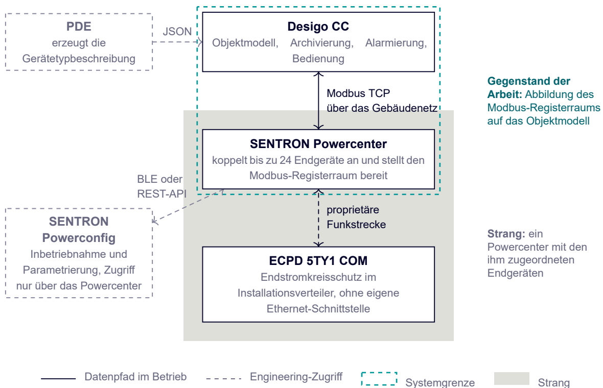
Abbildung 3: Datenpfad vom ECPD über die Funkstrecke zum Powercenter, von dort über Modbus TCP im Gebäudenetz zu Desigo CC, seitlich angetragen die Werkzeuge SENTRON Powerconfig und PDE mit ihren jeweiligen Zugriffspunkten
