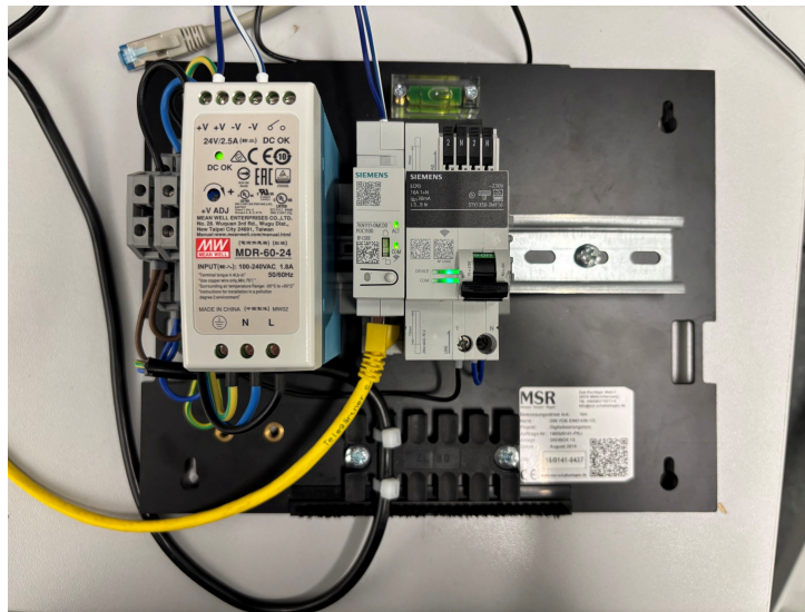
Abbildung 5: Laboraufbau aus 24 V Netzteil, Powercenter 1100 und ECPD 5TY1 COM
