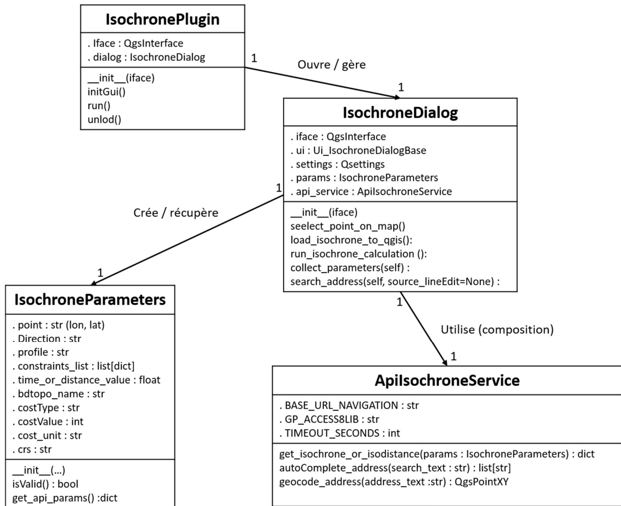
Figure : Diagramme de classe
