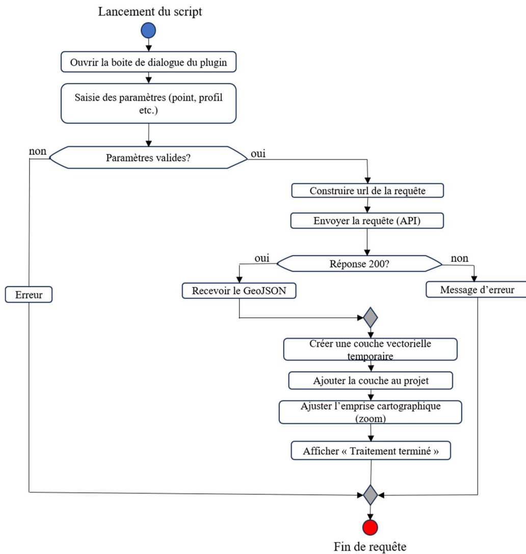
Figure 2 Diagramme de cas d'activité
