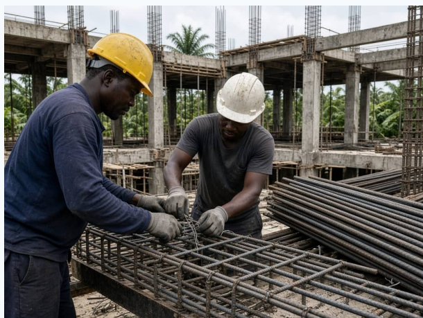
Ferraillage poutres R+3
