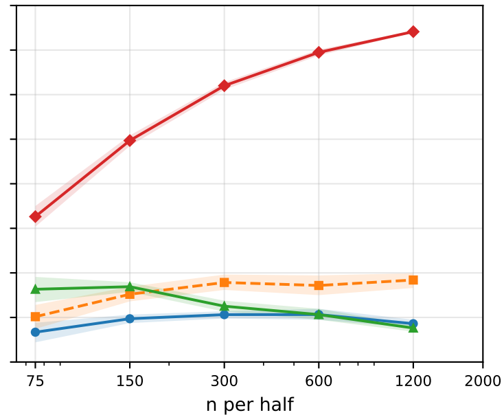
Llama-3-8B-abl, layer 21 (focus)
