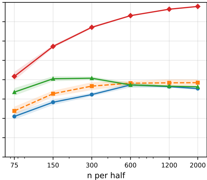
Qwen3.6-27B, layer 54
