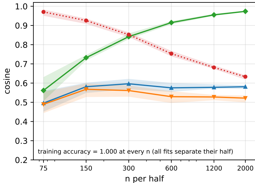
Qwen3.6-27B, layer 43
