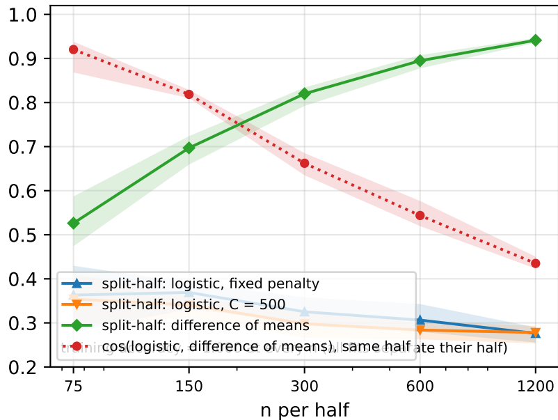
Llama-3-8B-abl, layer 21
