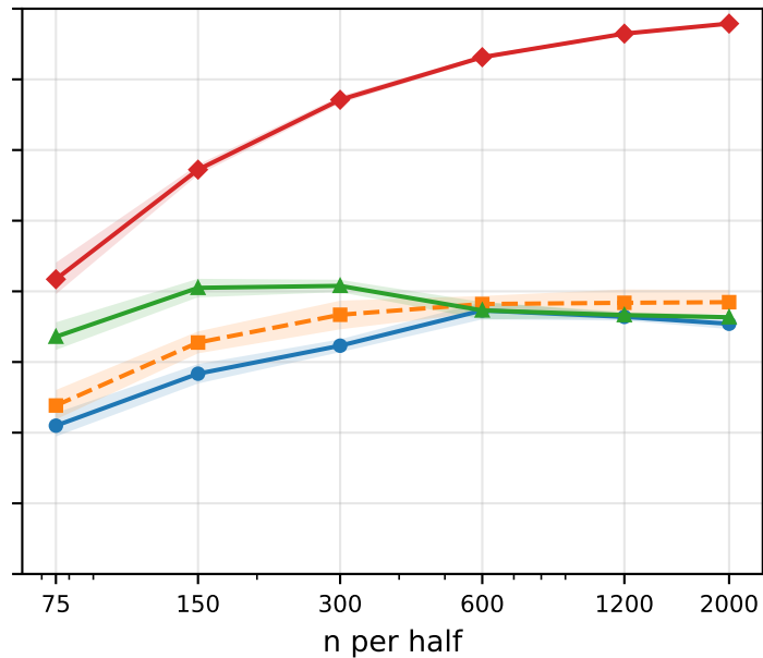
Qwen3.6-27B, layer 54
