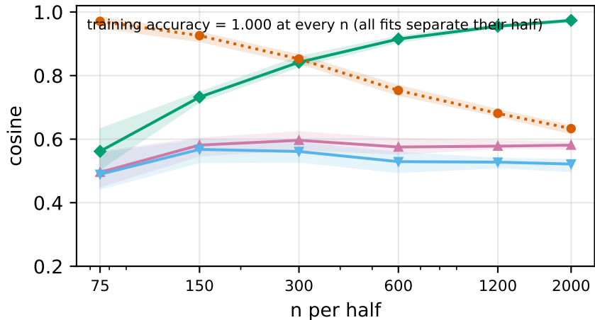
Qwen3.6-27B, layer 43
