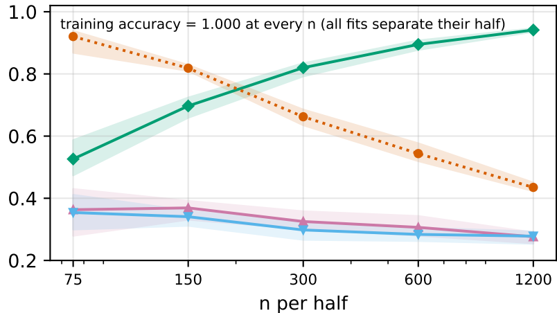
Llama-3-8B-abl, layer 21
