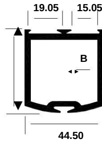
Door vertical plain
