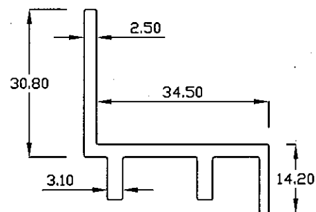
14013 0.602 Kg/m
