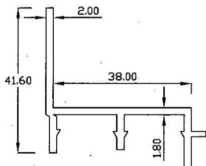
14024 0.527 Kg/m
