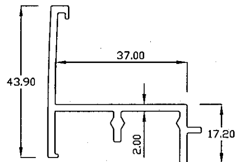
14027 0.610 Kg/m
