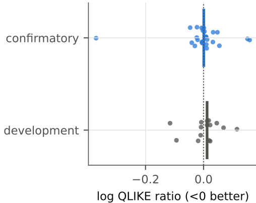
H2: Analogue+HAR vs HAR
