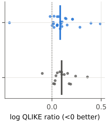
H3: Analogue vs HAR
