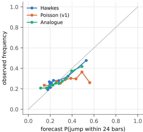
BTC — tail-risk calibration (OOS)
