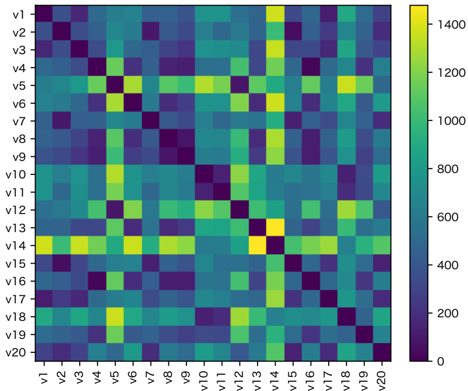
マンハッタン距離行列
