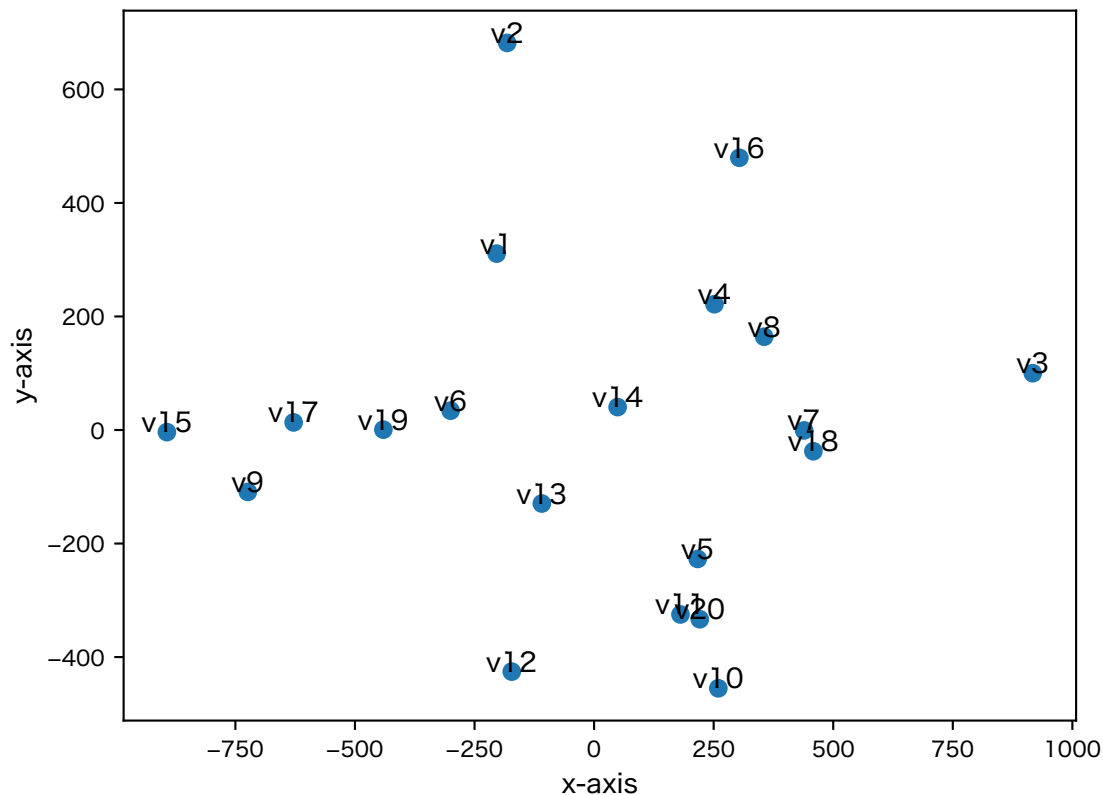
距離に基づく2次元埋め込み (MDS)
