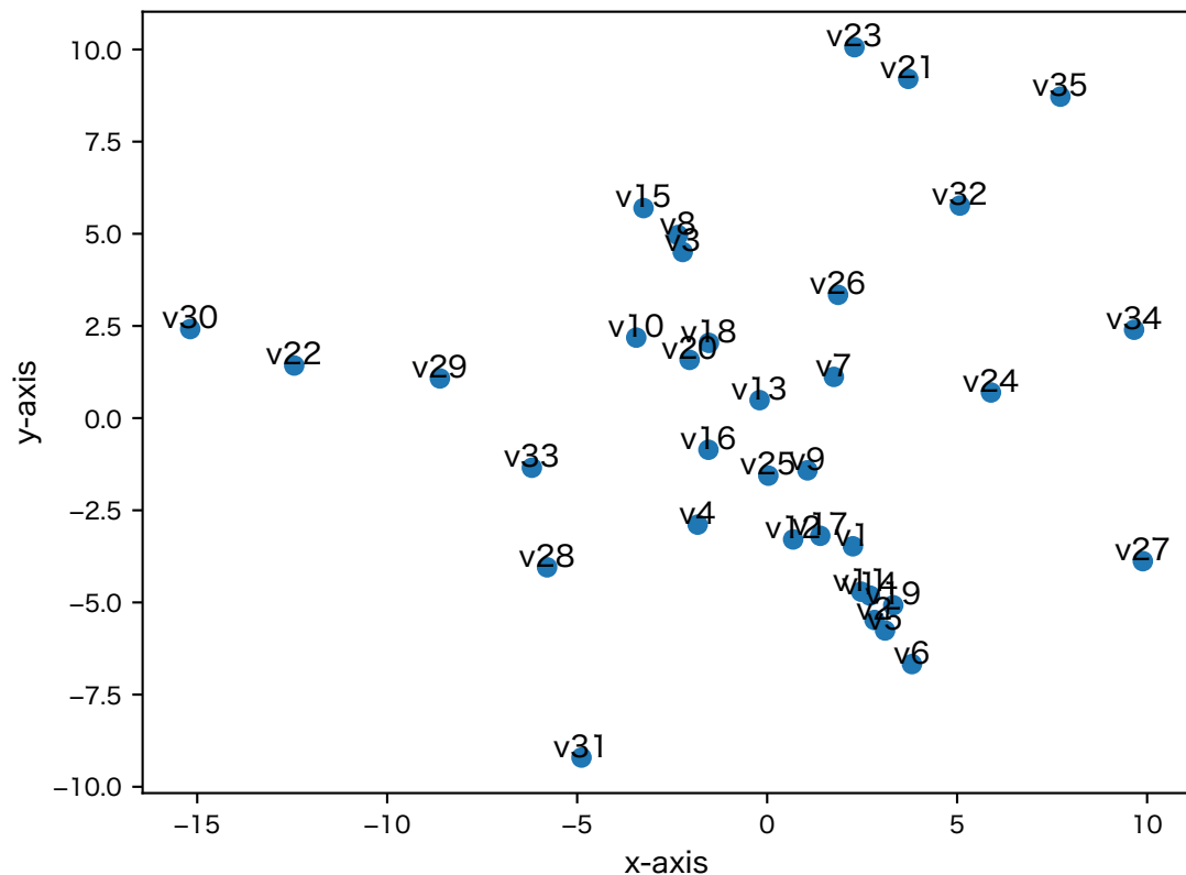
距離に基づく2次元埋め込み (MDS)
