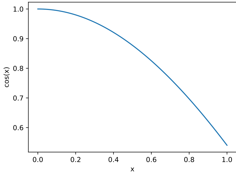
\cos(x)
