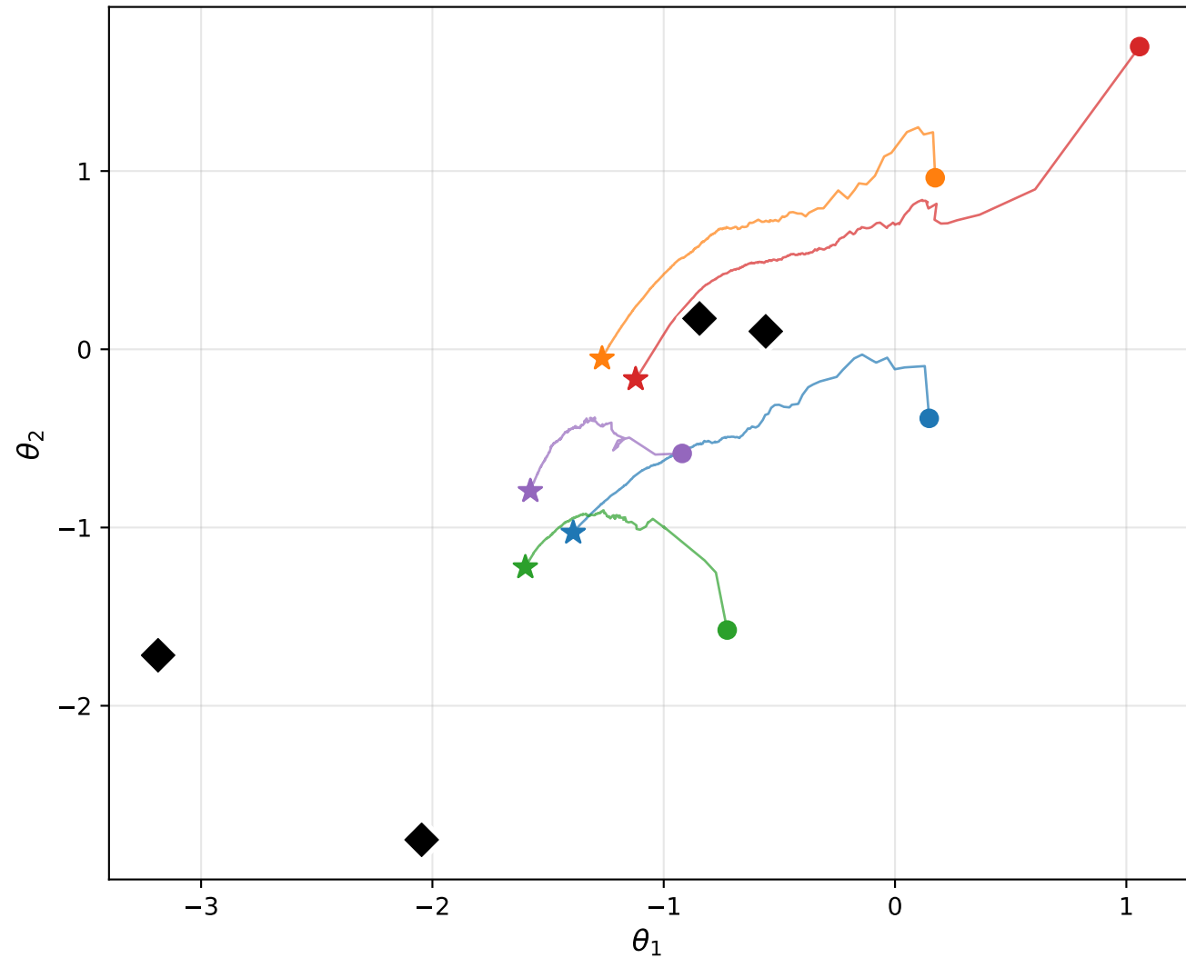
Parameter Space (Worst Policy MDP)
