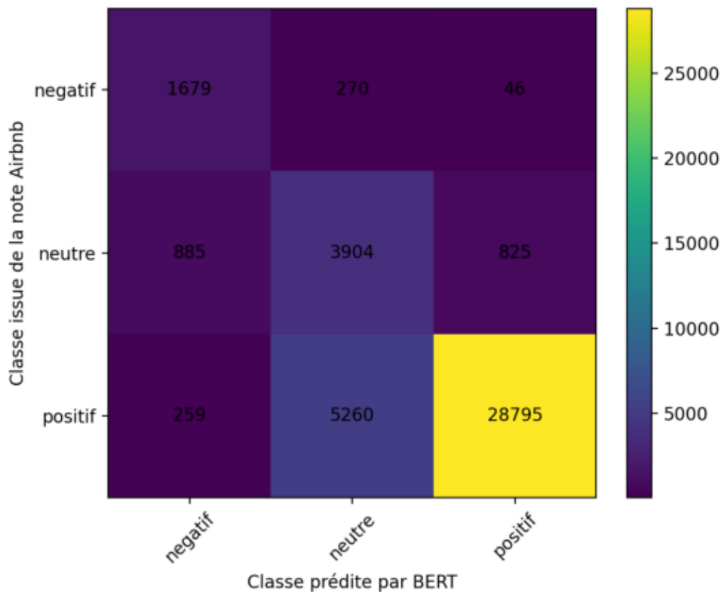
Matrice de confusion : classes note Airbnb vs classes BERT
