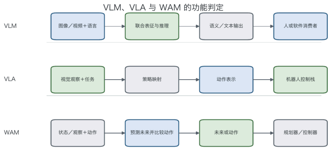
三条泳道分别列出视觉—语言模型、视觉—语言—行动模型和世界动作模型的输入、机制、输出和消费者。
