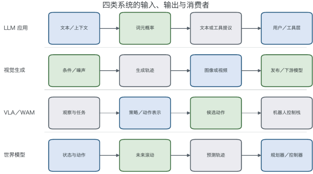
四条横向泳道分别展示语言模型、视觉生成、视觉语言行动系统和世界模型的输入、内部过程、输出与消费者。
