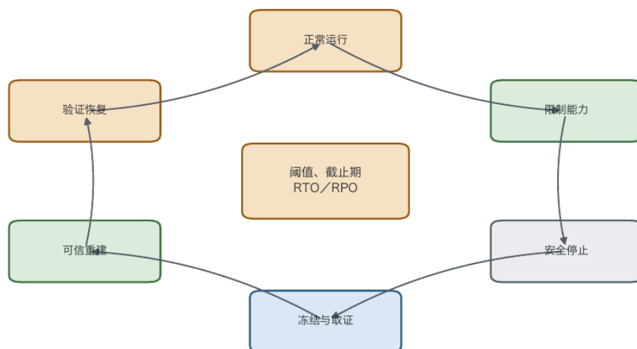
从异常发现到验证恢复的状态机
