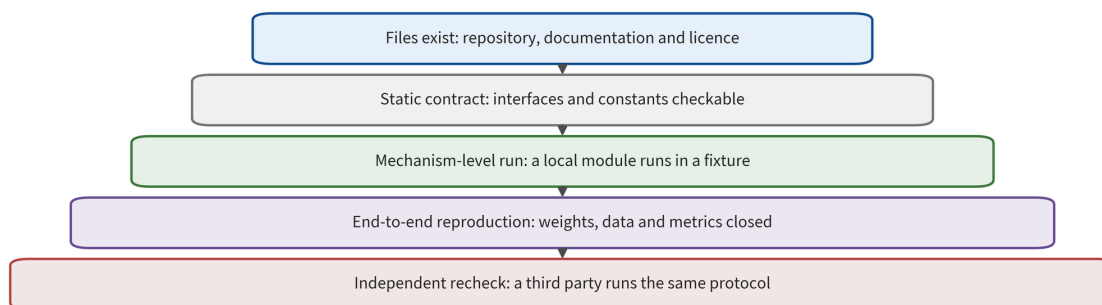
F10 Reproduction maturity ladder
