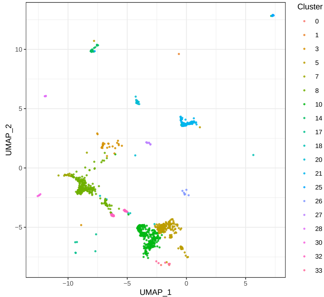
UC01/current 12049: global Seurat cluster
