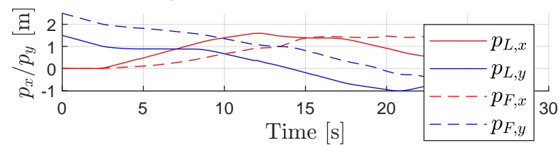
Coordinates evolution
