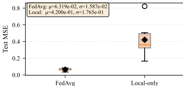
(d) Distribution of per-client test MSE
