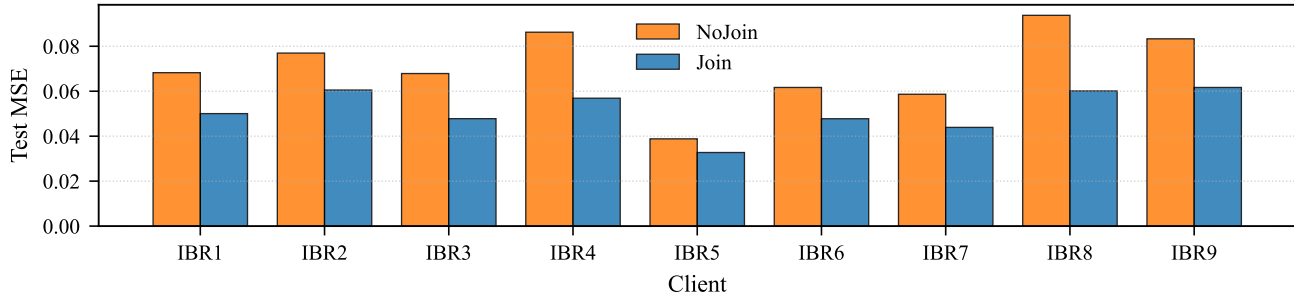
Per-client test MSE
